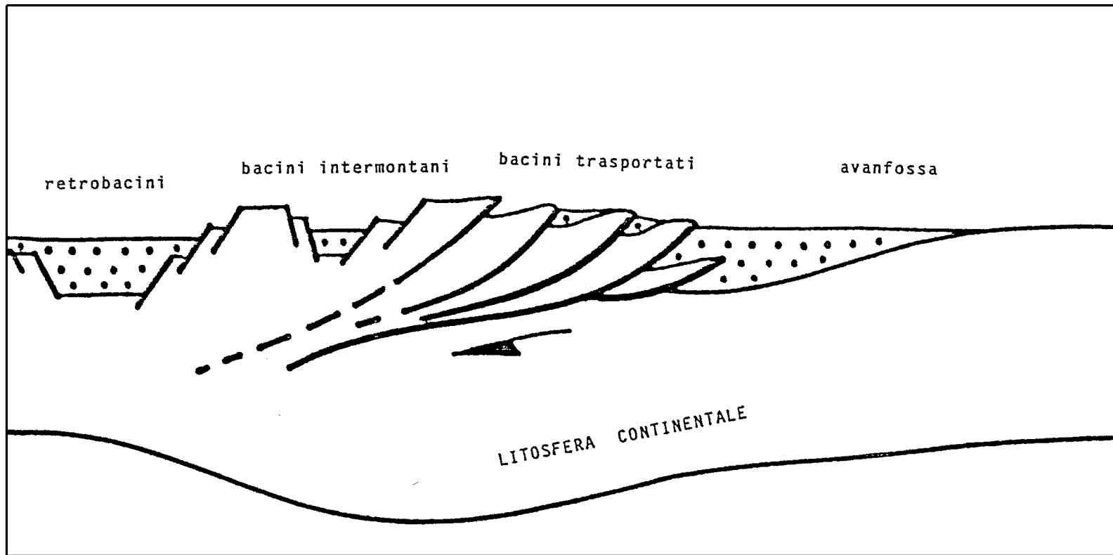
Fig. 3 - Sistema post-collisionale appenninico. (Ricci Lucchi e Ori, 1985).
